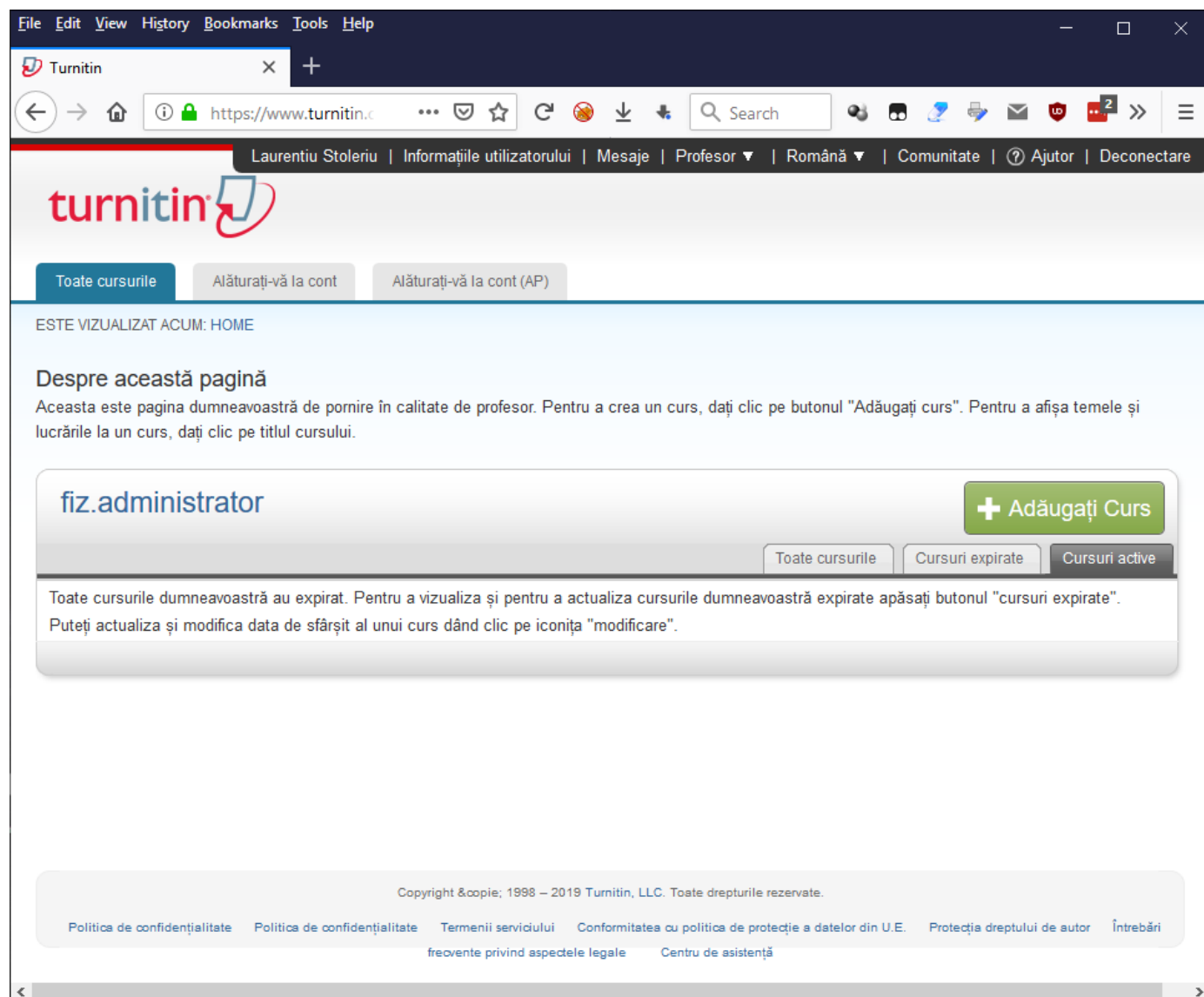
Fig. 2 – Pagina inițială.
