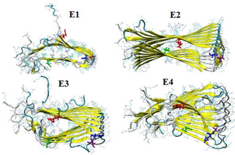
Figura V.9. Modelele simulate E1-E4 ale oligomerilor de amilină după înlăturarea legăturilor disulfidice Cys2-Cys7
