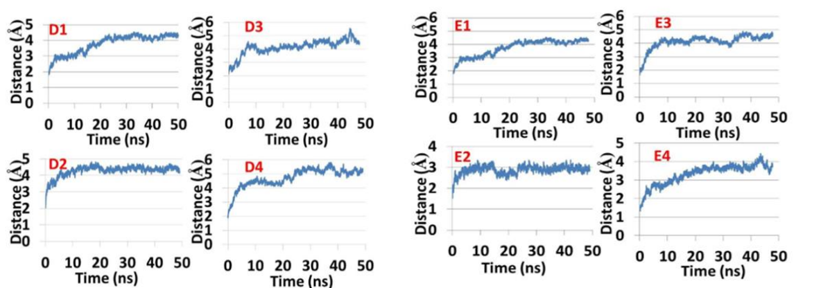
Figura V.14 & V.15.. Analiza RMSD pentru modelele D1-D4 și E1-E4
