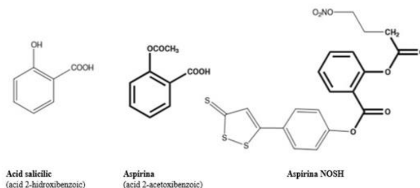
Figura V.21. Formula chimică a aspirinei NOSH
